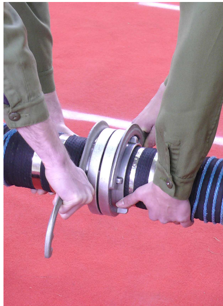
Abb.8b: Ansetzen der Kupplungsschlüssel und das Kuppeln der Saugschläuche
