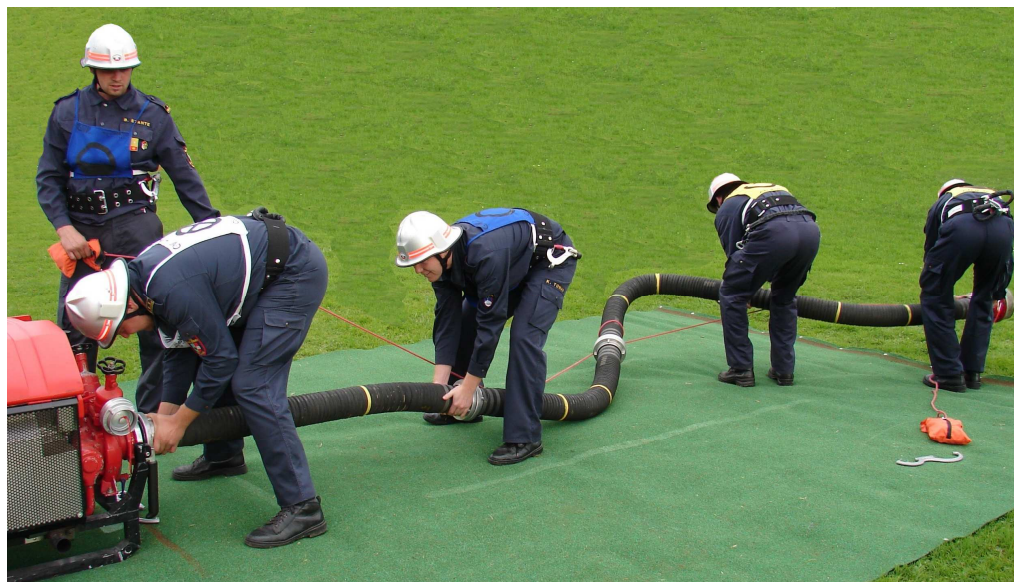
Abb. 14: Ankuppeln der Saugschlauchleitung an die Tragkraftspritze
