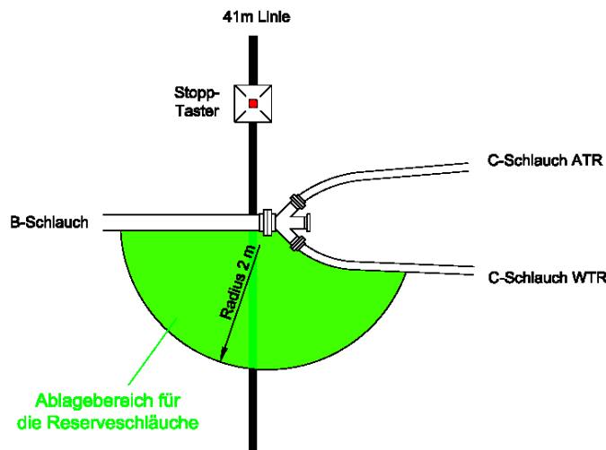
Abb.19 Richtiges Ablegen der Reserveschläuche
