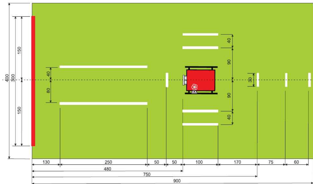
Abb.1: Bodenmarkierung für das Aufstellen der Bewertungsgeräte
